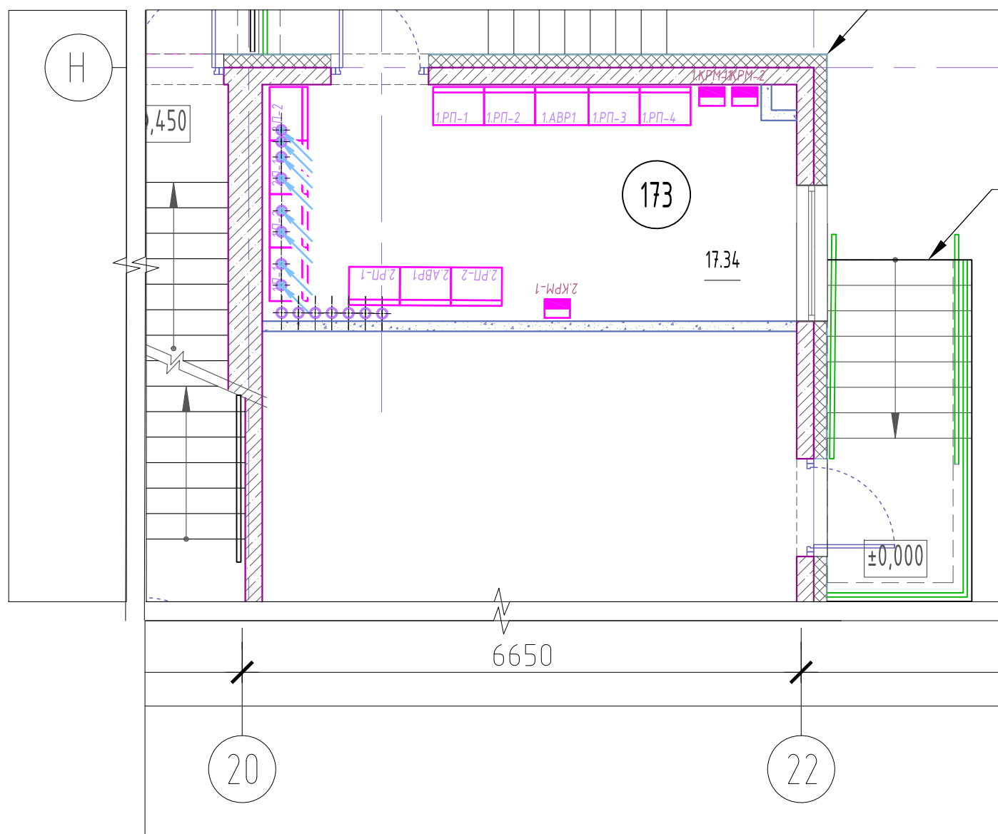
План расположения силовых щитов ВРУ
