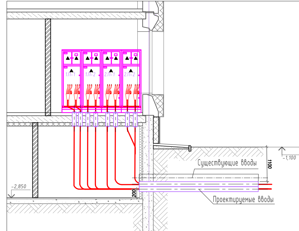
Разрез 1-1
